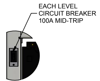
(1:8)A DETAIL
