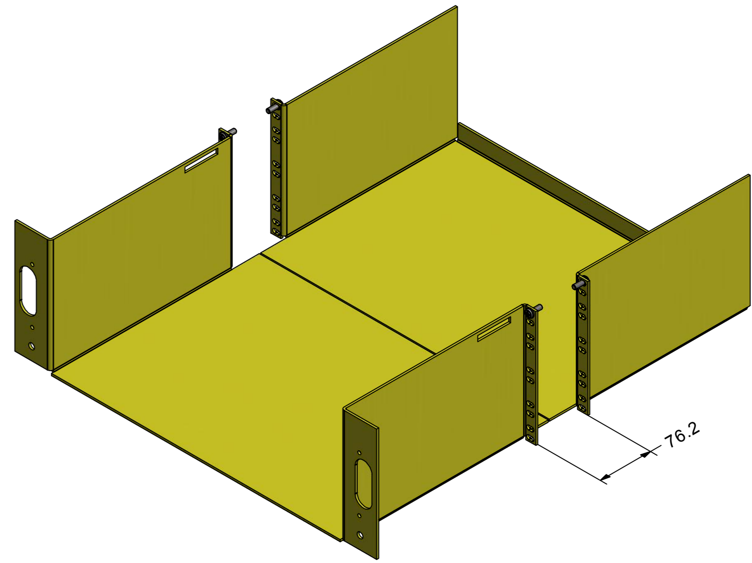
ISOMETRICO
